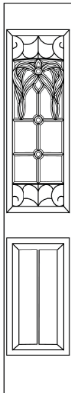
1'2" x 6'9" 1/2 Lite Sidelight
